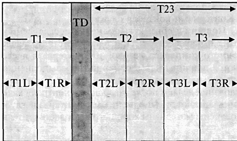
Рисунок 1. Наименования, размеры и расположение треков в формате API для вывода первичных кривых ГИС на твердые носители
